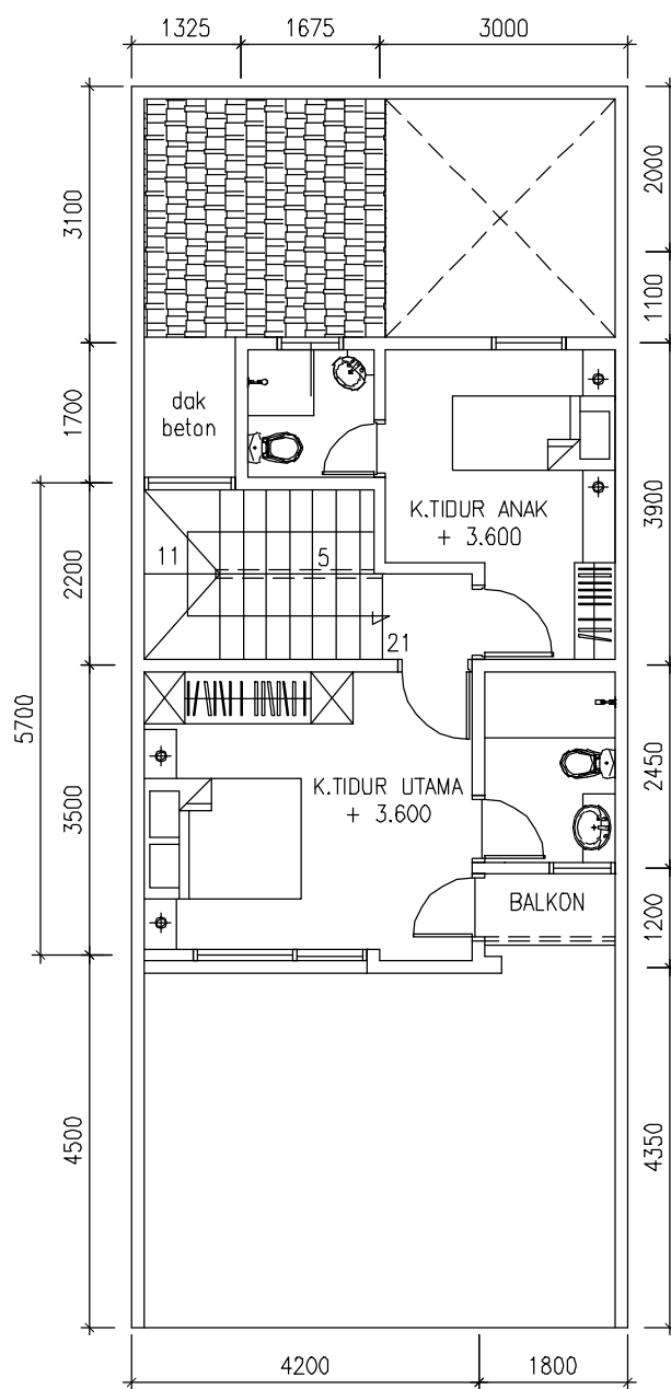
— — DENAH LT. ATAS TYPE 84/90 SCALE 1 : 50
